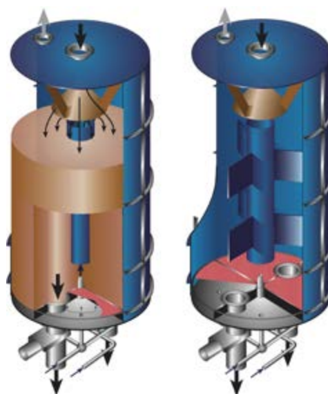
НР Гомогенизатор.
