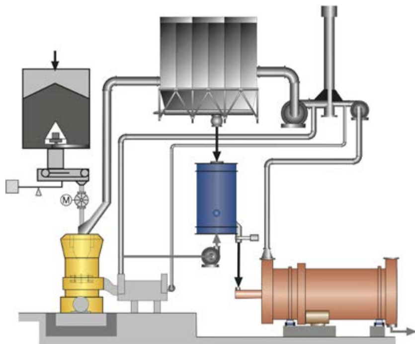
Кальцинация синтетического гипса в горизонтальном ударном кальцинаторе.
