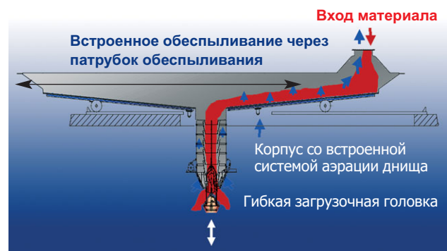
Принцип загрузки и обеспыливания
