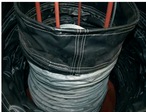
Загрузочное устройство с внешним и внутренним складчатыми рукавами для стандартных материалов (например, цемента)
